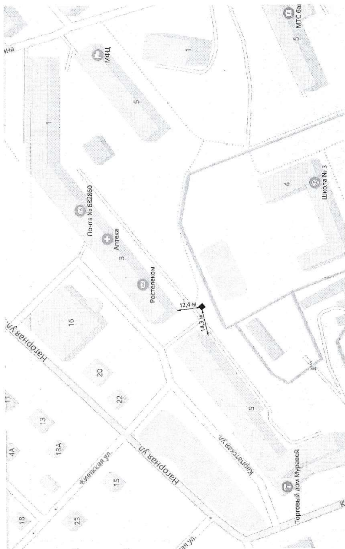
Схема размещения места (площадки) твёрдых коммунальных отходов № 17
