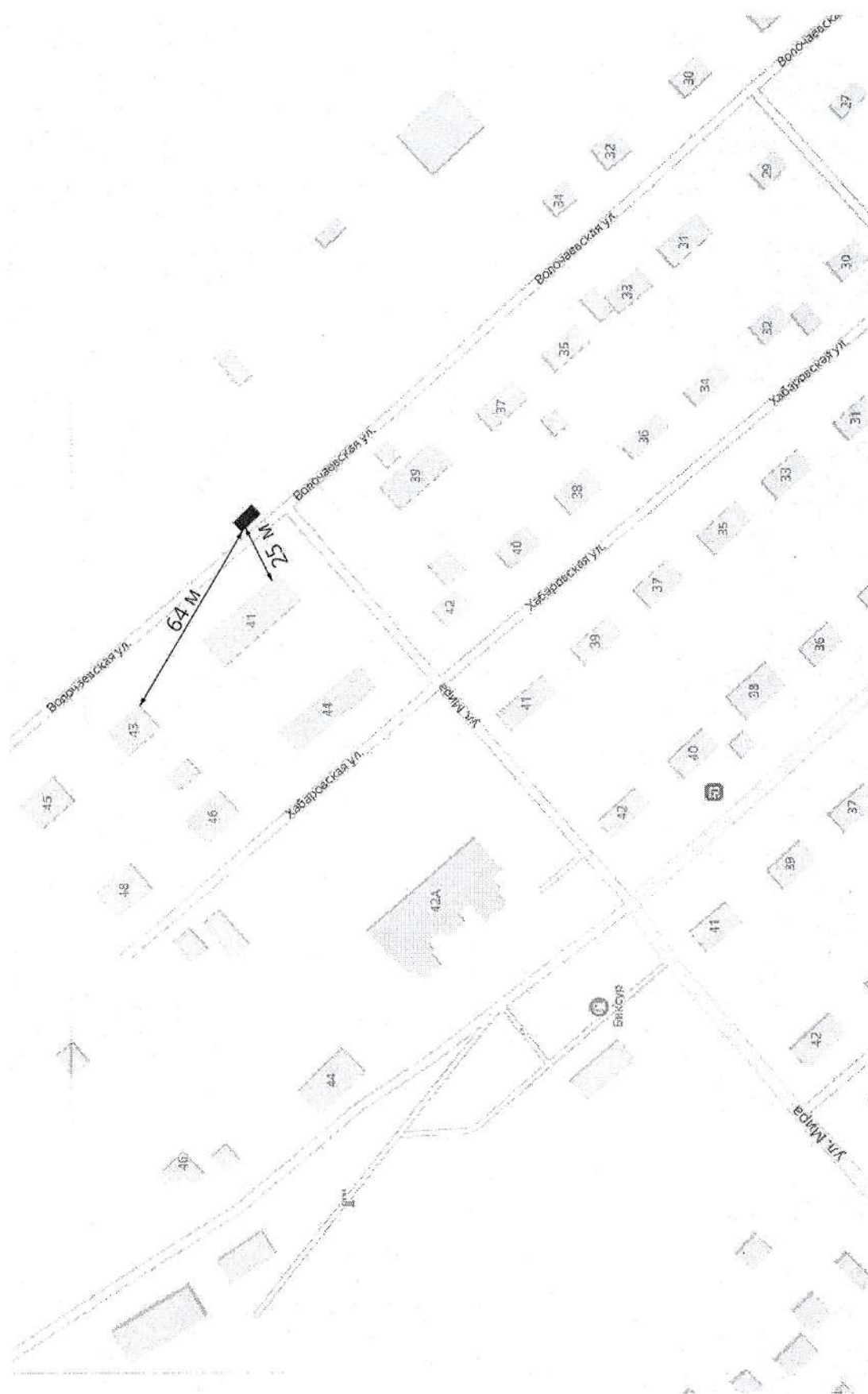
Схема размещения места (площадки) твёрдых коммунальных отходов № 35
